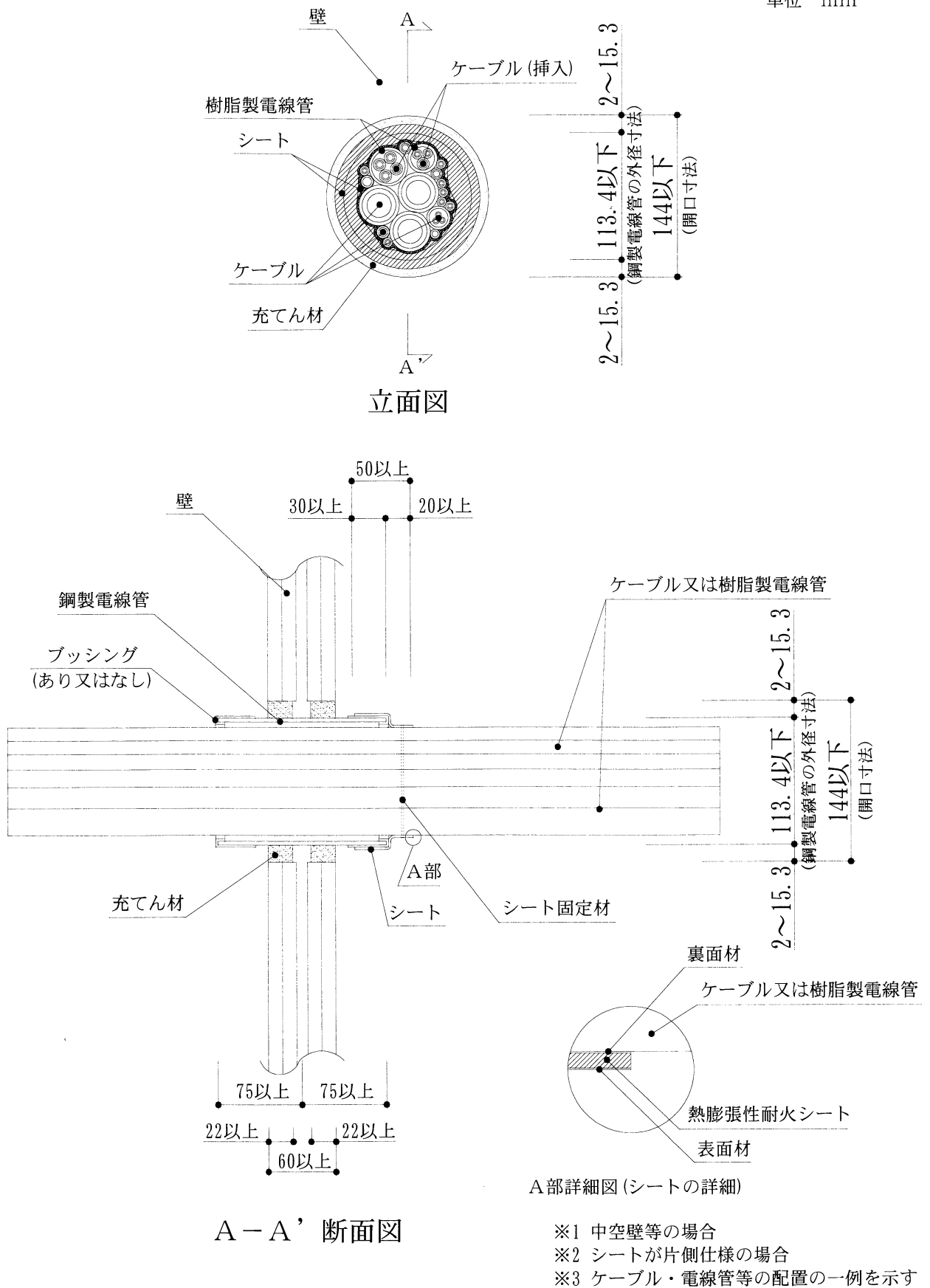
図1 構造説明図 (施工図)
