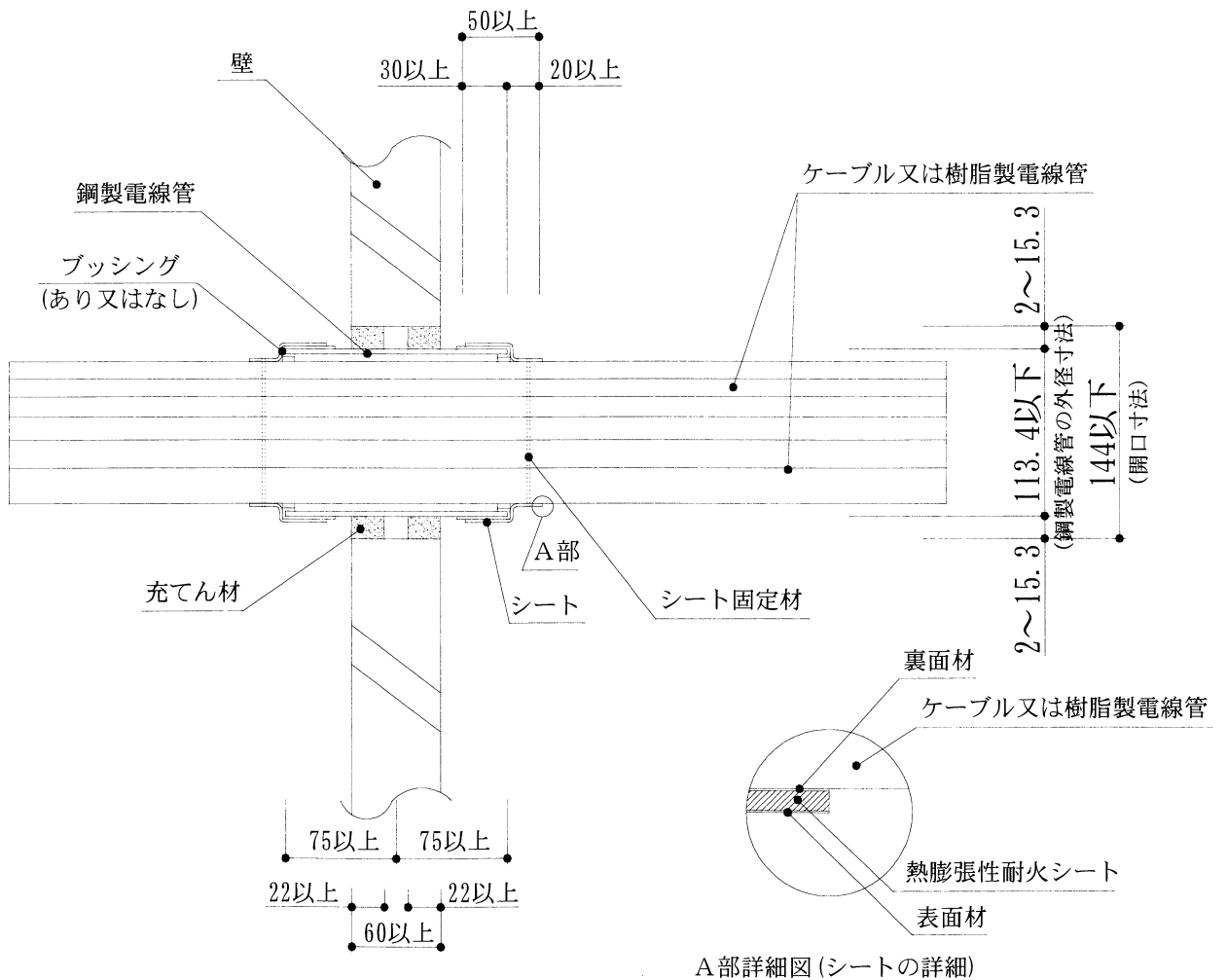
A-A' 断面図
